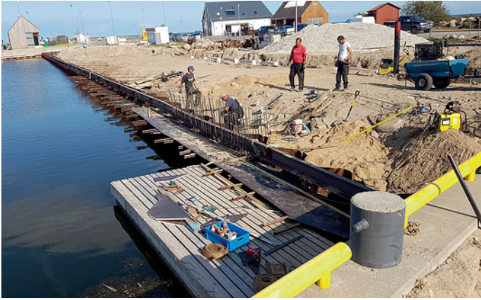
Sulund on sees, algavad betoneerimistööd. Pildil Kihnu Majanduse OÜ ehitusbrigaad
